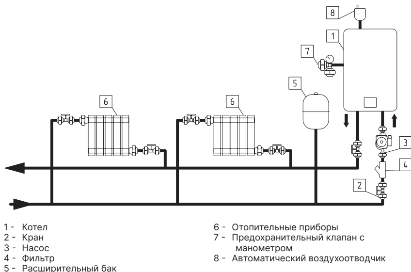
Схема 1 «Подключение - подача и обратка снизу, предохранительный клапан в резьбовое отверстие сбоку, воздухоотводчик сверху»
