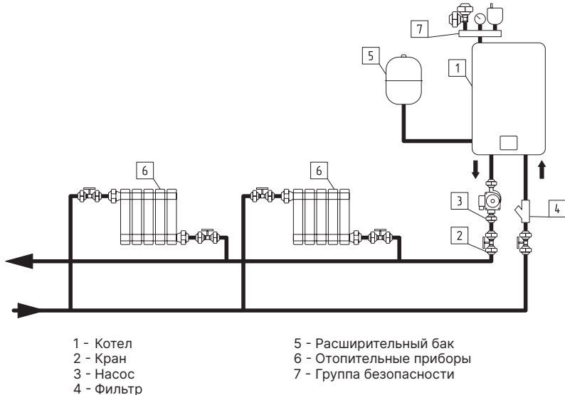
Схема 2 «Подключение - подача и обратка снизу, группа безопасности с воздухоотводчиком сверху, расширительный бак в резьбовое отверстие сбоку»
